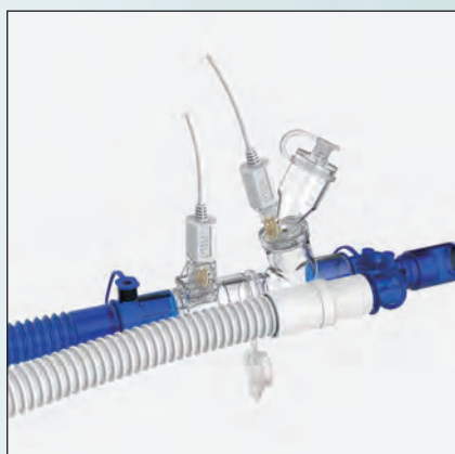
薬液カップ+エアフローセンサの 呼吸回路への接続例(吸気側)
